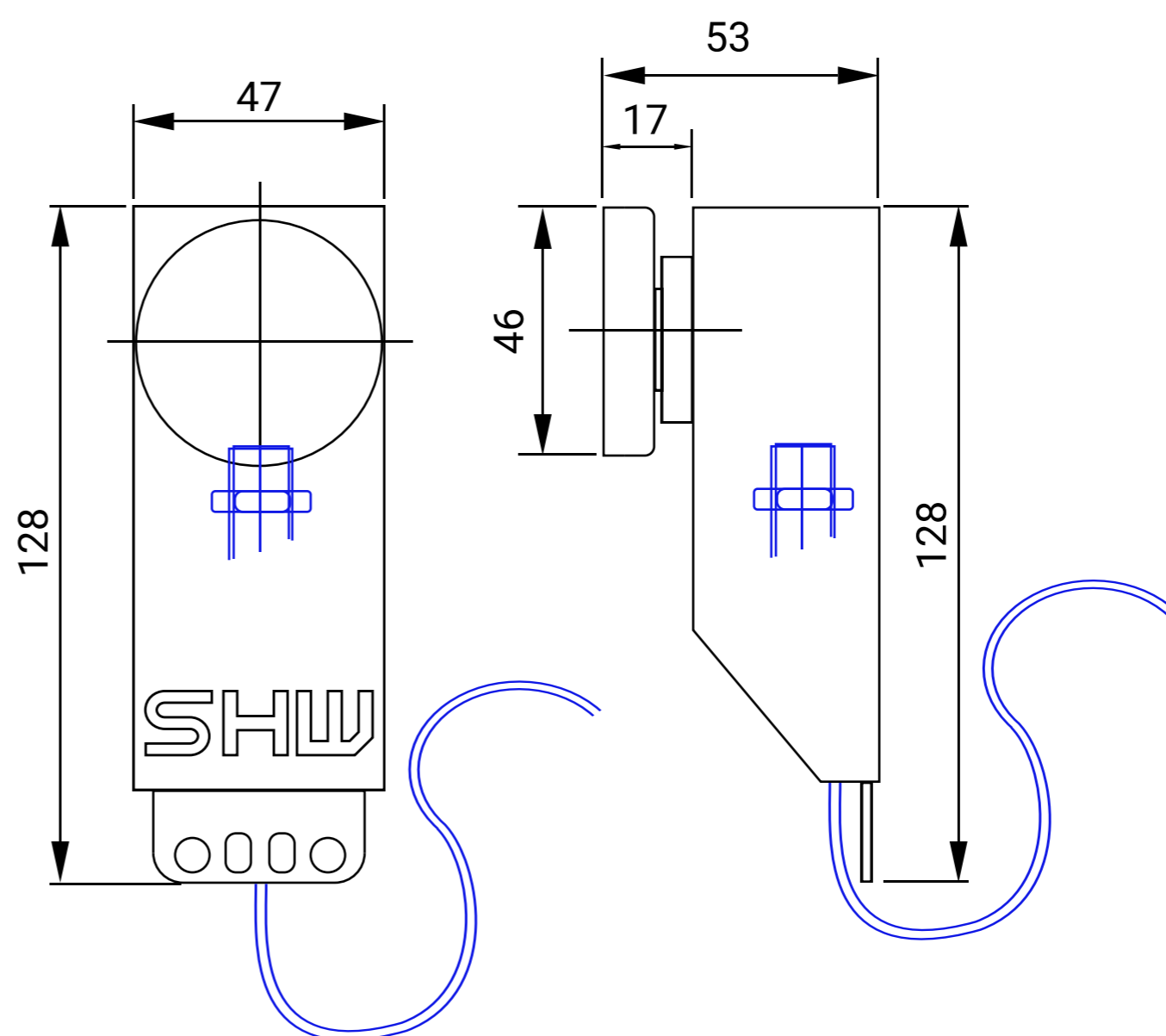
Medidas dimensionais
